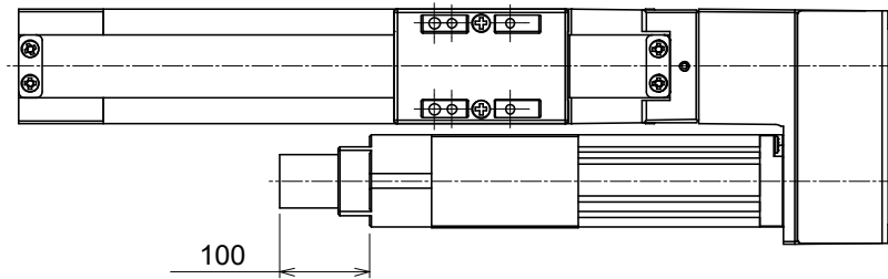
b) RCA2-SA2AR
